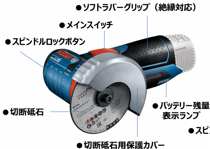
コードレスカッティングディスクグラインダー GWS 10.8V-76H (本体のみ)
