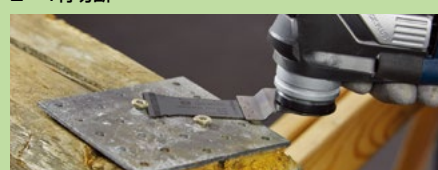
ビス面一切断
