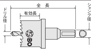
■寸法図
